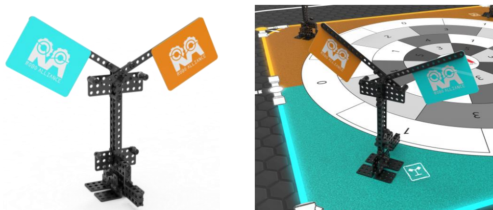
图 2.31 “活动旗台”初始状态及其放置位置
