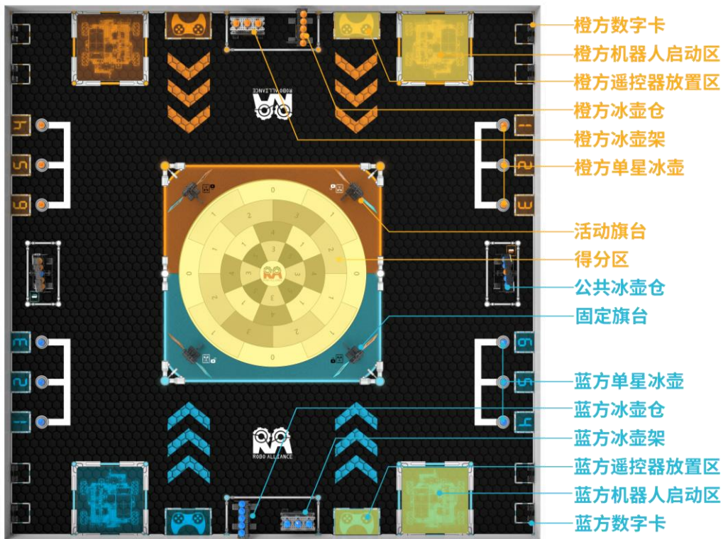
图 2.39 比赛场地分布
